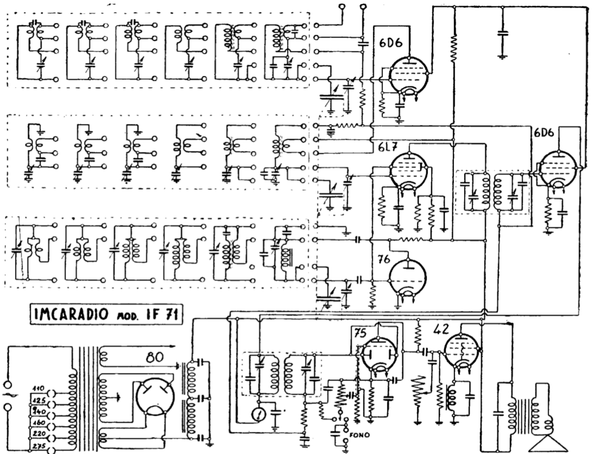
59. — IMCARADIO. — Mod. « IF 71 ». — Produzione 1937. — Media frequenza: 467 kHz.
